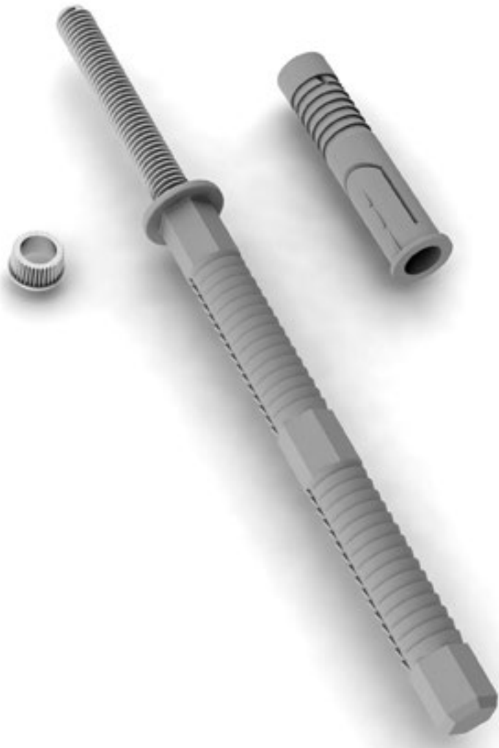
Suporte invisível para prateleira
