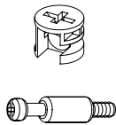
KIT COMPLETO C/ 50 PARAFUSOS E TAMBORES MINIFIX
